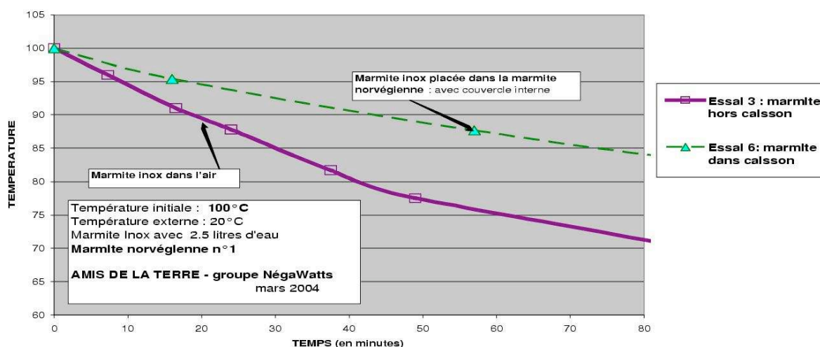
PERTE DE TEMPERATURE - TEST MARMITE NORVEGIENNE : mars 2004
